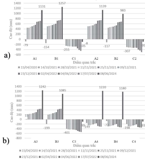
Hình 9. Cao độ xung quanh kè theo thời gian: a) MC 1 và MC 2; b) MC 3 và MC 4
