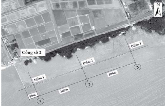
Hình 4. Sơ họa mặt bằng vị trí quan trắc độ lún của kè [7]
