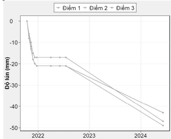
Hình 10. Kết quả quan trắc lún phần bê tông của kè ly tâm
